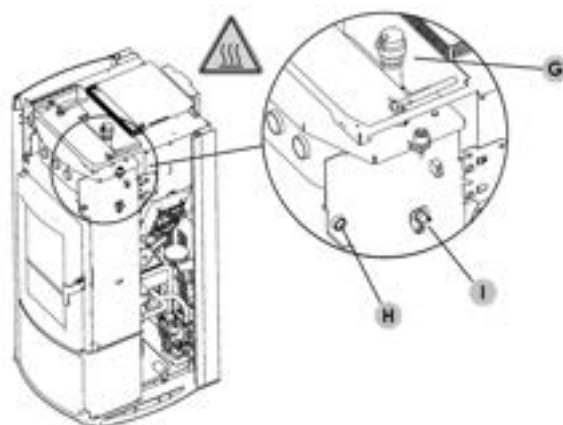
Fig. 39 - Purgeur manuel (situé sous le couvercle) (Idro Prince 3 16-23-23 H2O, Aquos 3 16-23-23 H2O, Idron 16-22 Airtight, Hidrofire 22.8)
