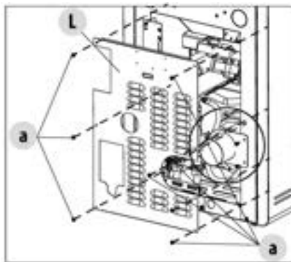
Fig. 51 - Panneau arrière
