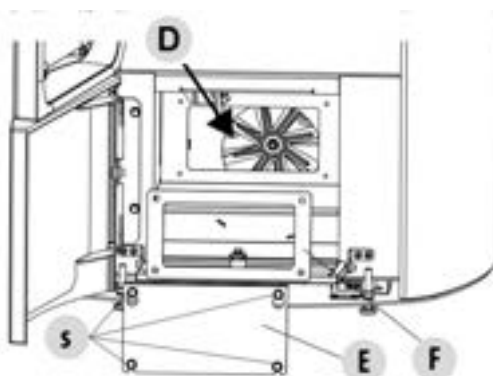
Fig. 55 - Nettoyage du compartiment inférieur
