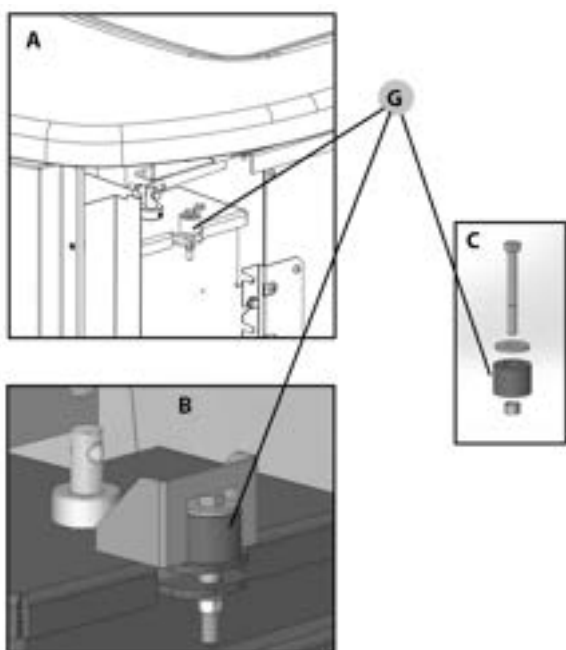
Fig. 66 - Caoutchouc
