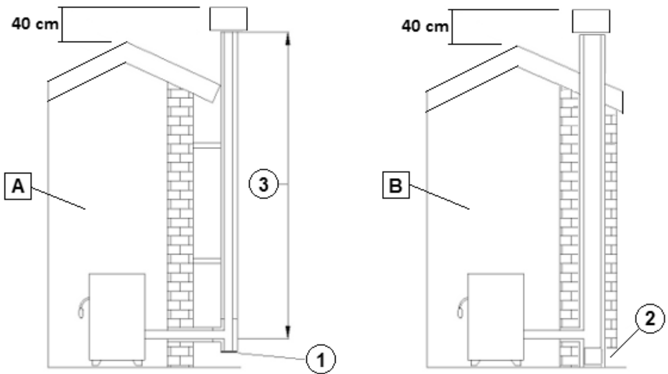
Fig. 6 - Conduit de fumées
