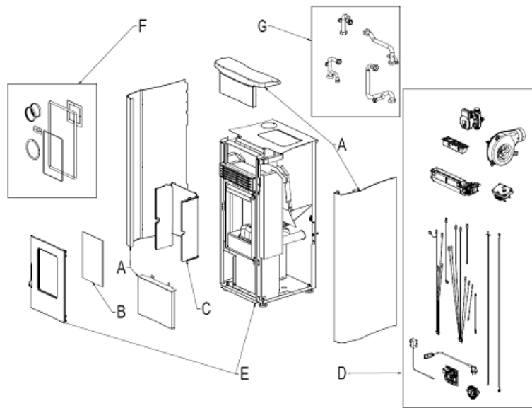
Fig. 1 - Dessin éclaté
