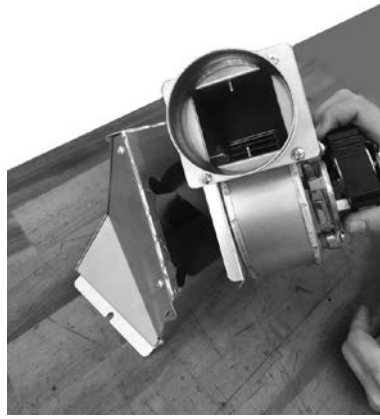
Fig. 41 - Fixer le ventilateur au carter
