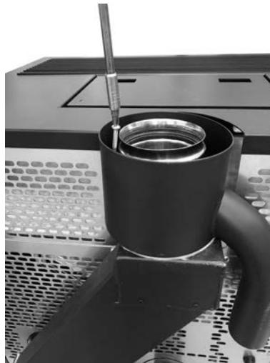
Fig. 50 - Fixer le concentrique sur le tuyau
