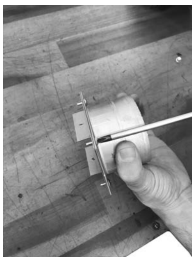
Fig. 37 - Fixer la bride au raccord
