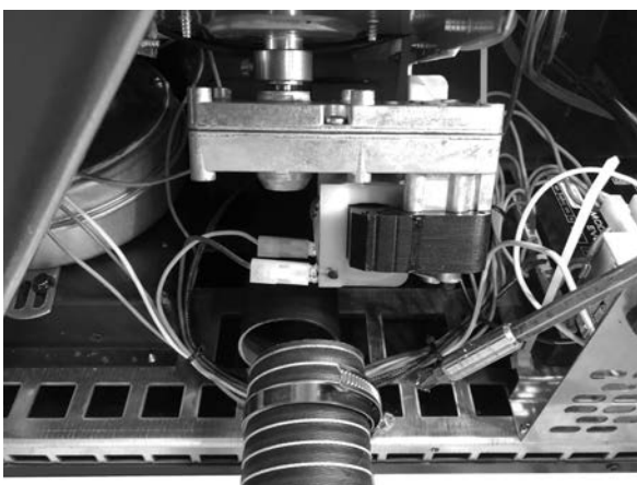
Fig. 52 - Branchement 2 entrées
