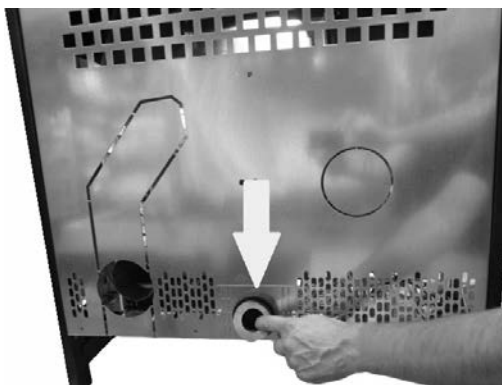
Fig. 33 - Extraction anneau
