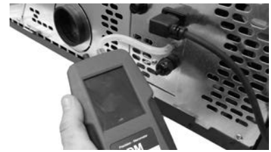
Fig. 59 - Connexion du pressostat numérique Modo At et Quasimodo 3 Up
