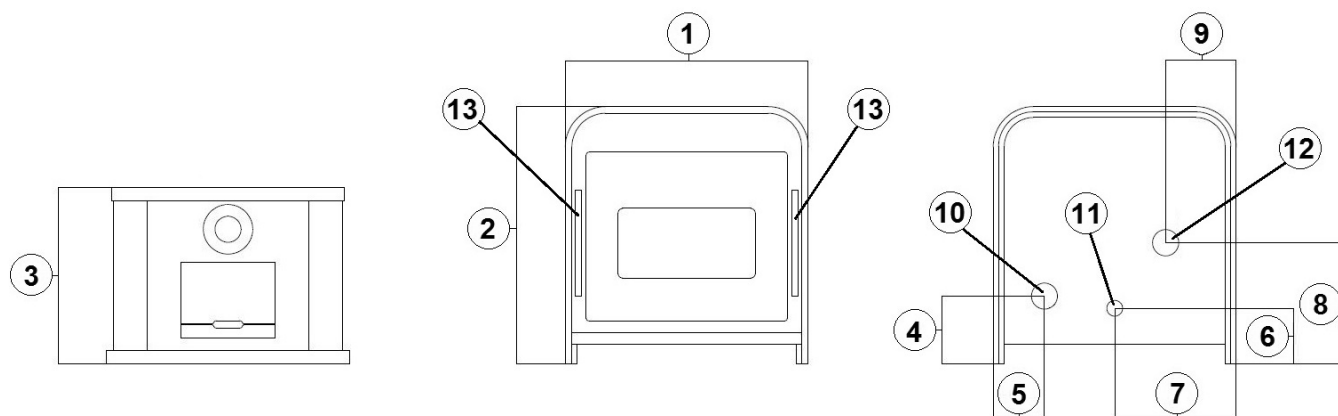
Fig. 20 - Dimensions générales: FRAME 3
