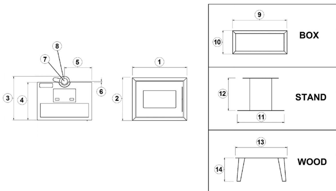
Fig. 23 - Dimensions générales: MODO AT
