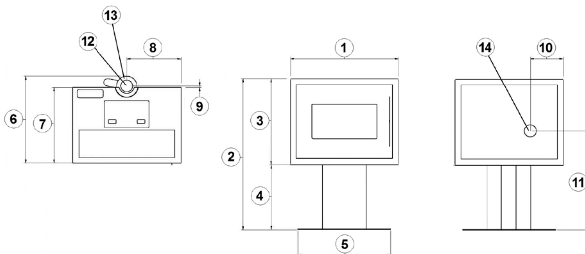
Fig. 22 - Dimensions générales: QUASIMODO³ UP
