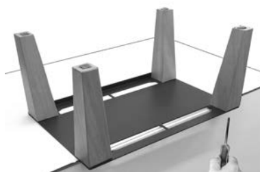
Fig. 26 - Fixer les pieds à la base
