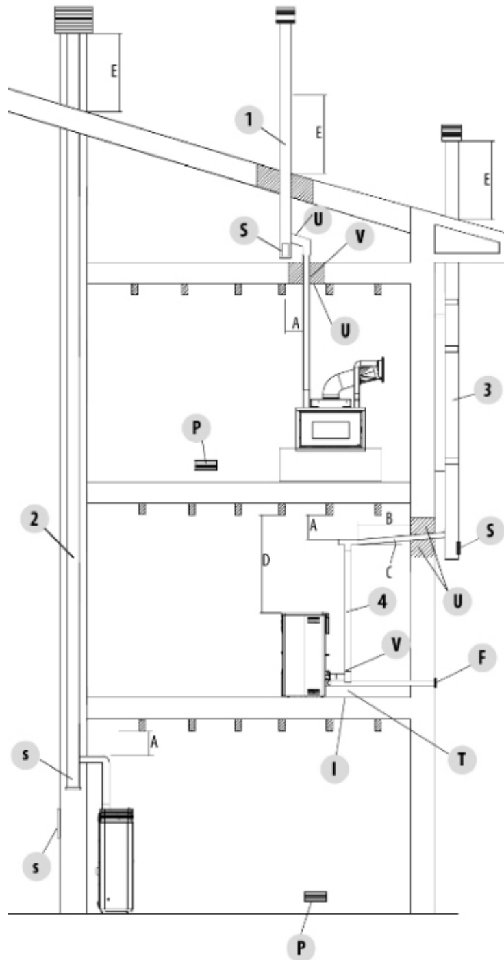
Fig. 10 - Conduit des fumées
