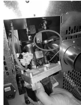
Fig. 62 - Retrait du motoréducteur
