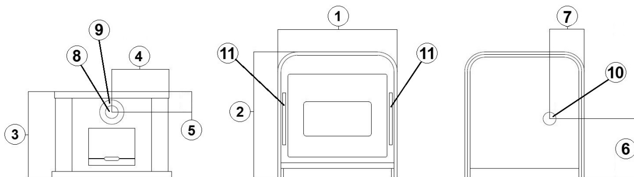
Fig. 21 - Dimensions générales: FRAME 3 UP
