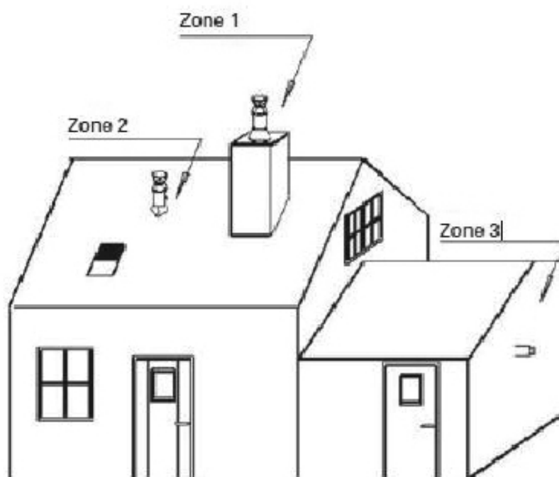
Fig. 11 - Définition des zones d'implantation
