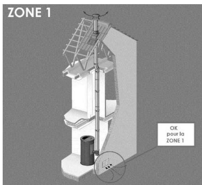
Fig. 14 - Installation possible pour tous les poêles (ZONE 1)
