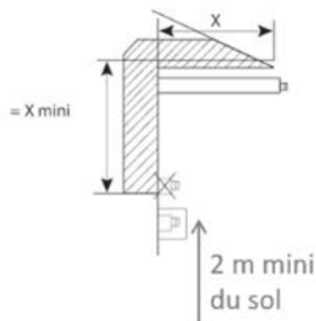
Fig. 13 - Rebord de toit
