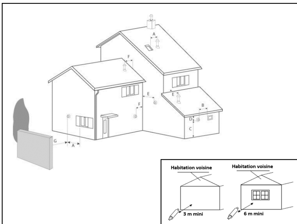
Fig. 12 - Position des terminaux
